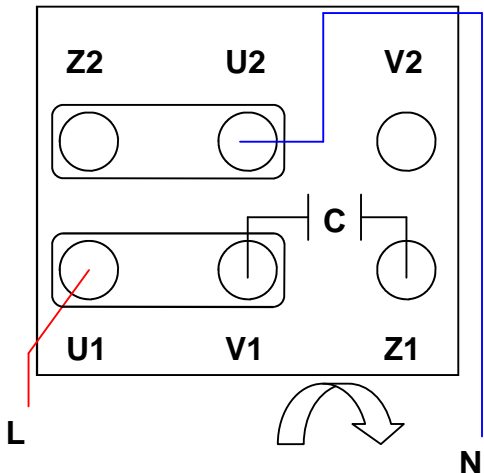
1 Phase 230 V
